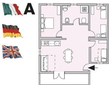
Tipo A: 3 camere + soggiorno (6+2) Typ A: 3 Schlafzimmer + 1 Wohnzimmer (6+2) Type A: 3 bedrooms + living-room (6+2)
