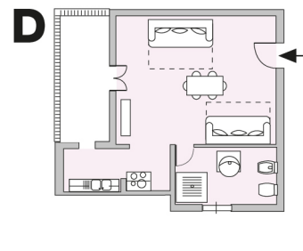
Tipo D: monovano / soggiorno (4) Typ D: Schlafzimmer + 1 Wohnzimmer (4) Type D: bedrooms + living-room (4)
