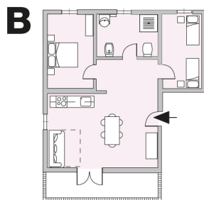
Tipo B: 2 camere + soggiorno (4+2) Typ B: 2 Schlafzimmer + 1 Wohnzimmer (4+2) Type B: 2 bedrooms + living-room (4+2)
